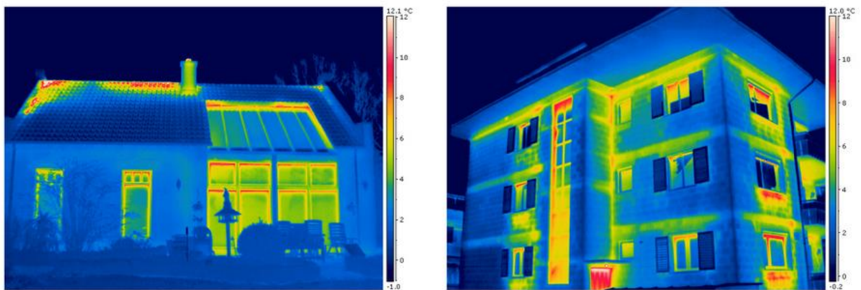
Beispielbilder der Thermografieaufnahme eines Einfamilienhauses (links) und eines Mehrfamilienhauses (rechts).
